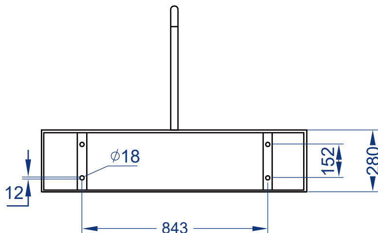
安装底座图
