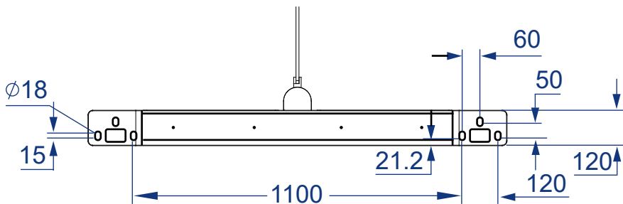
安装底座图
