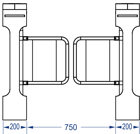
正视图
