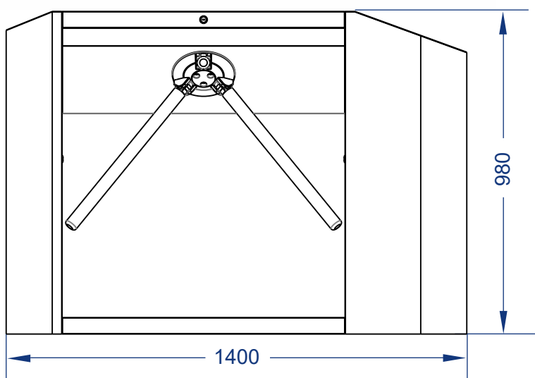
侧视图
