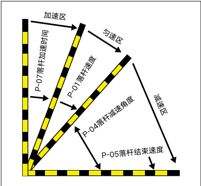
4. 无低速运行区的落杆示意图 (P-26 等于 0)
