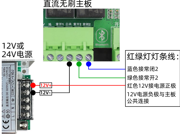
P-44 红绿灯接线图
