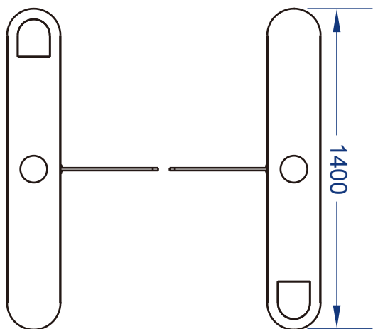
俯视图
