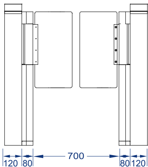
正视图
