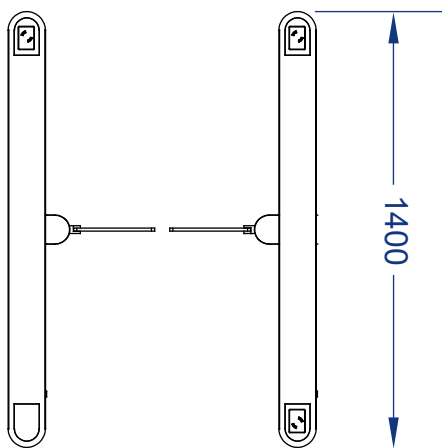
俯视图
