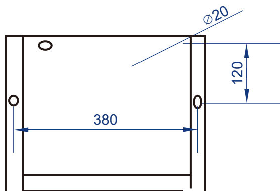
安装底座图
