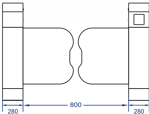
正视图
