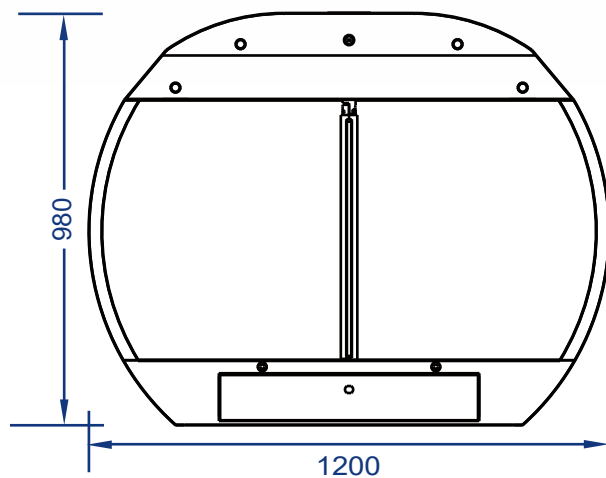
侧视图
