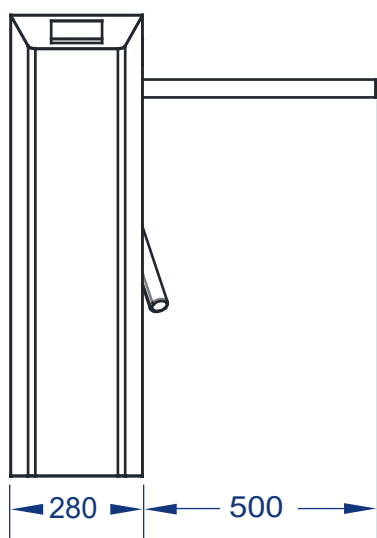
正视图
