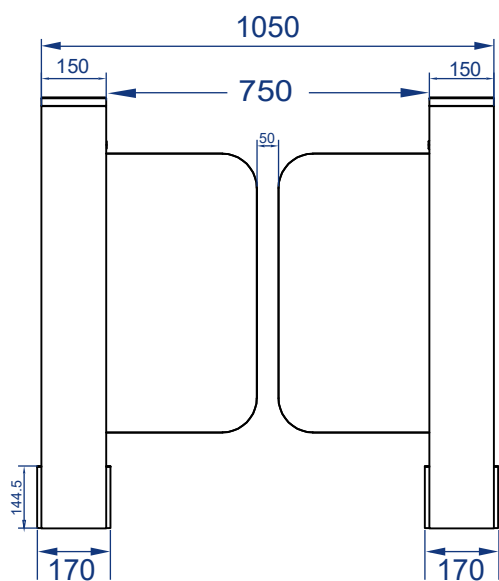
正视图
