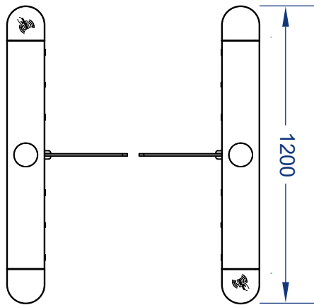
俯视图
