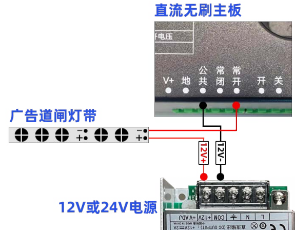
P-44 红绿灯接线图
