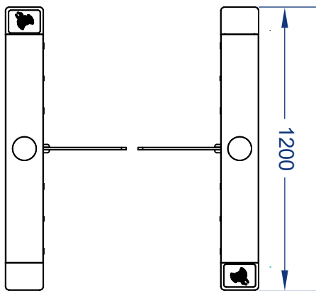
俯视图
