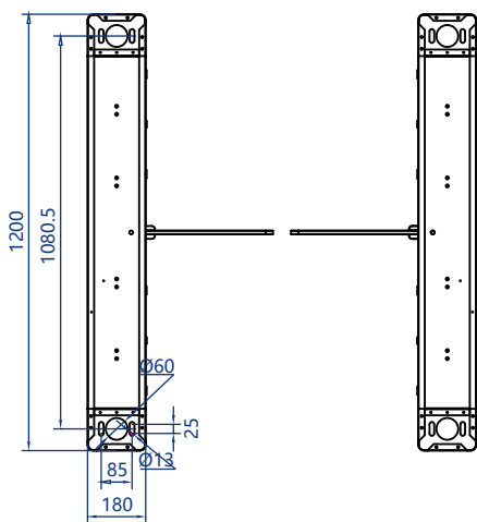
安装底座图
